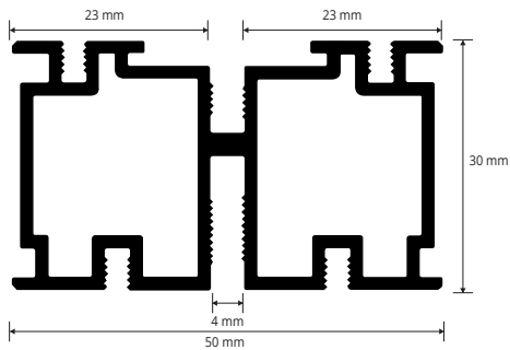
PRORAIL - RAIL PREFORMÉ aluminium - Cond. 10 Pce. - Longueur b. 2,7 ML
