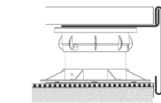
PROSUPPORT B - PROFILO TOP - ALLUMINIO VERNICIATO lunghezza barre 2,7 ml - conf. 10 Pz (PFPSAL...1060 conf. 20 Pz)
