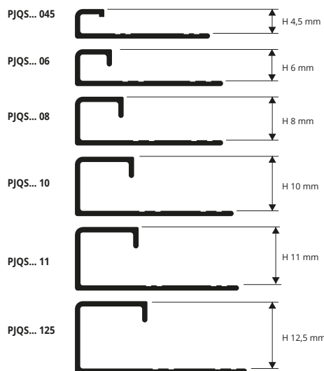
ALL. ANODIZZATO thermo packed (argento-oro-rame-titanio-nero) lung. barre 2,7 ml - conf. 40 PZ - 108 ml (H 12,5 mm - conf. 20 Pz - 54ml)
