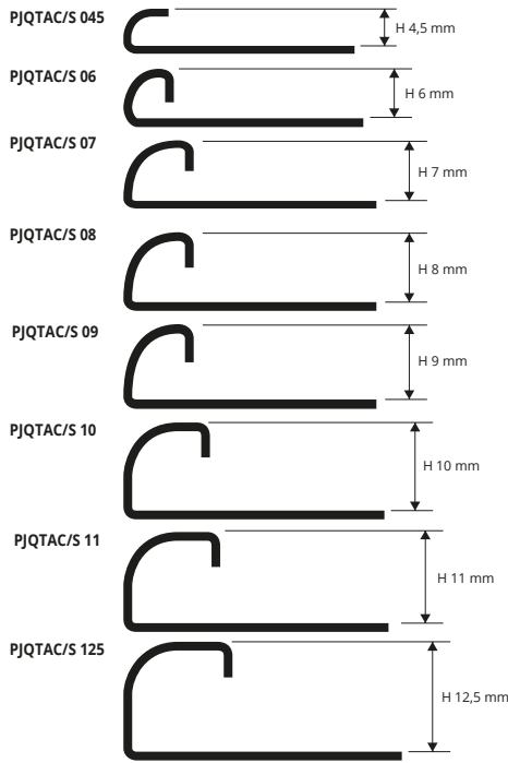
EDELSTAHL AISI 304/1.4301-V2A GLÄNZEND mit Schutzfolie Stangenlänge 2,7 Lfm VE 20 Stk. - 54 Lfm (H 4,5 mm - 108 Lfm) - 10/10 mm
