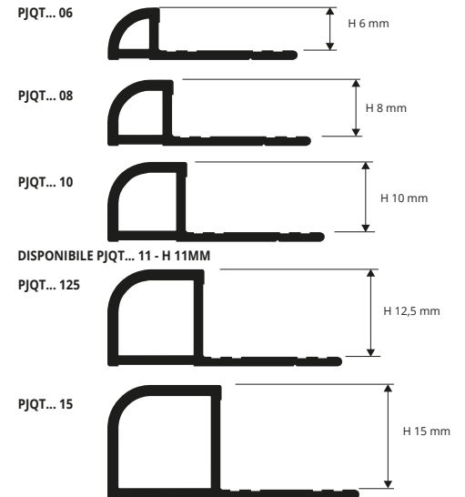
ALU. GLÄNZEND (Chrom, Titan und Gold) Thermoverpackung - Stangenlänge 2,7 Lfm - VE 40 Stk. - 108 Lfm (H 12,5-15 mm - VE 20 Stk.)
