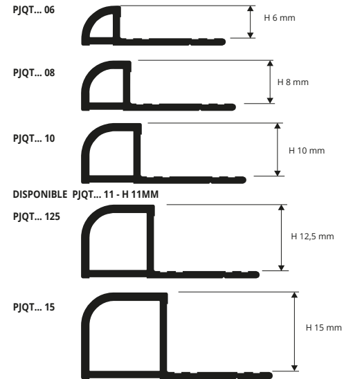
ALUMINIUM BRILLANTÉ thermo packed - longueur b, 2,7 ML cond. 40 Pcs - 108 ML - (H 12,5 mm, 15 mm - cond. 20 Pcs)
