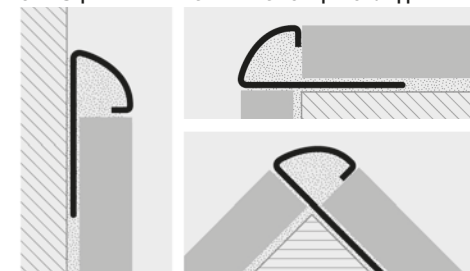
ПЕСКОСТРУЙНАЯ НЕРЖАВЕЮЩАЯ СТАЛЬ AISI 304/1.4301-V2A - длина бруска 2,7 ЛИН.М упак. 20 шт. - 54 ЛИН.М - 10/10 мм
