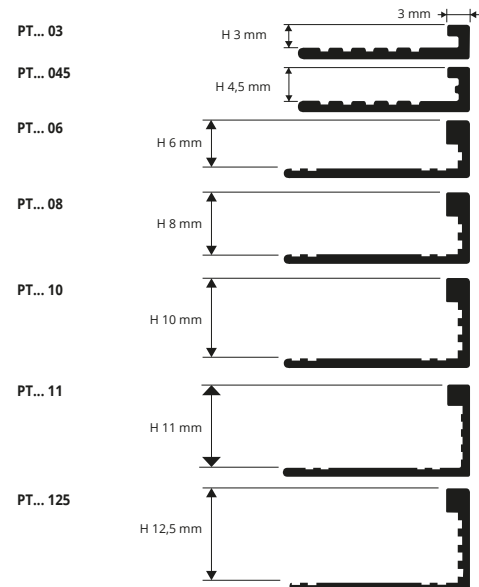
АНОД. АЛЮМ. отделка титан, медь, чёрная, бронза и бронза с эфф старения в термоупаковке - длина бруска 2,7 Лин.М - упак. 40 шт. - 108 Лин.М
