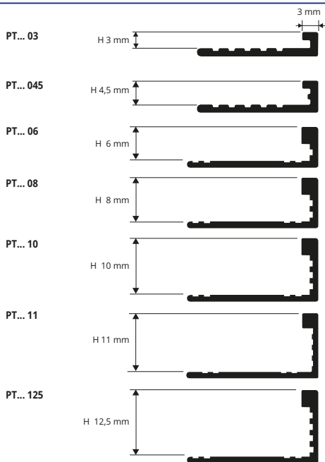
ALUMINIO BRILLANTE (cromo, titanio, negro, oro, cobre) termo empaquetado Unidades de 2,7 M de largo - Paq. de 40 UD - 108 M
