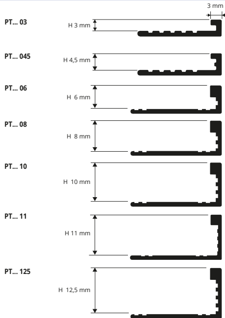
ALUMINIUM BRILLANTÉ (chrome, titane, noir, or et cuivre) thermo packed - longueur b. 2,7 ML - cond. 40 Pces - 108 ML
