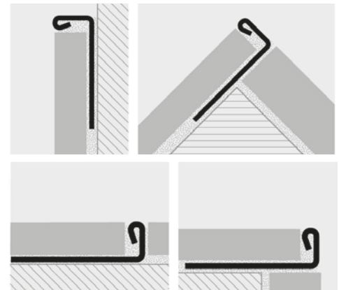
EDELSTAHL AISI 304/1.4301-V2A-V2A GLÄNZEND mit Schutzfolie Stangenlänge 1 Lfm - VE 40 Stk. - 40 Lfm - 10/10 mm
