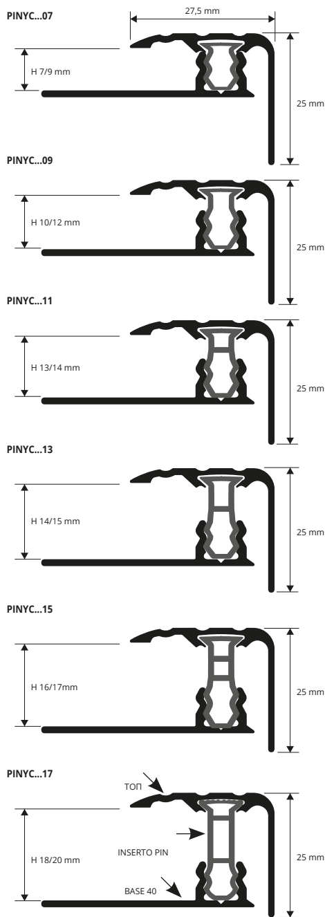
ТОП/ПРОФИЛЬ ИЗ АНОД. АЛЮМ.
