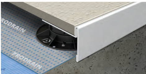
PROSUPPORT A - ALLUMINIO NATURALE TRANCIATO E FORATO lunghezza barre 2,7 ml - conf. 20 Pz
