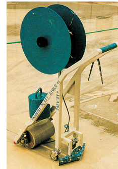
MÖRTELSCHLAMMSCHABER FÜR EINE GENAUERE VERLEGUNG
