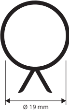
R 113 Maßstab 1:1
