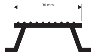
GCT 30 échelle 1:1
