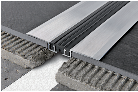
ALUMINIUM NATUR + EINSATZ AUS VINYLHARZ/GUMMI Stangenlänge 2,7 Lfm - VE 10 Stk. - 27 Lfm
