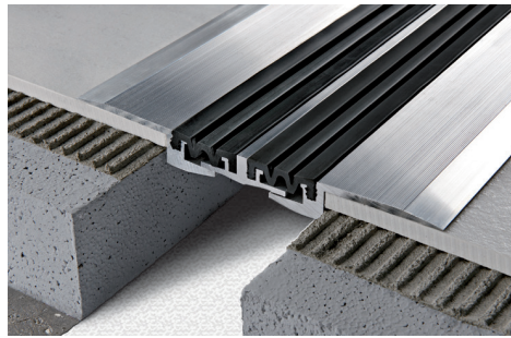
AUSWECHSELBAREM EINSATZ AUS VINYLHARZ / GUMMI SCHWARZ ODER GRAU - Stangenlänge 2,7Lfm - VE 10 Stk. - 27 Lfm
