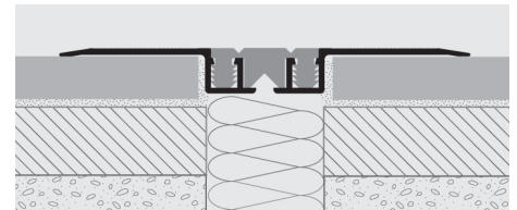
AUSWECHSELBAREM NEOPRENEINSATZ SCHWARZ ODER GRAU Stangenlänge 4 Lfm - VE 10 Stk. - 40 Lfm
