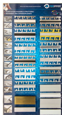
Pannello Campioni n° 10 Proflex, Prodilat, Giunti Posa Malta, Giunti Posa Colla
