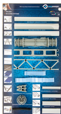
Pannello Campioni n° 18 Smussatura Triangolare, Rapy 100/200, Smusso Triangolare, Distanziatore Rigato, Prodistanz, Waterstop, Copritrefolo, Distanziatori PAU/PAV
