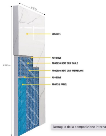
Stratigrafia del termoarredo Proheater
