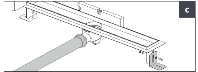
ABLAUFREDUZIERSTÜCK
