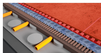
DISTRIBUTION DE LA CHALEUR
