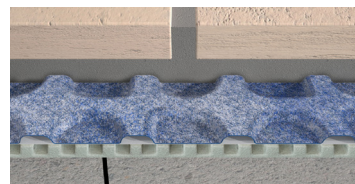
DESOLIDARISATION
