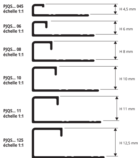
ALUMINIUM ANODISÉ thermo packed (argent-or-cuivre-titane-noir) longueur b. 2,7 ML - cond. 40 Pcs - 108 ML (H 12,5 mm - cond. 20 Pcs - 54 ML)
